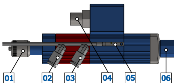
Figura 01 – Dettaglio DAV 200 – DAV 200
