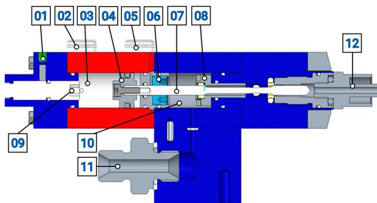
Figura 03 – Sezione interna DAV 200
